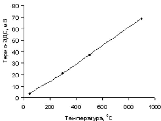
Рисунок 1 – График зависимости термо-ЭДС от температуры
